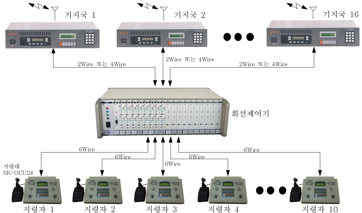
그림1 시스템 구성도
